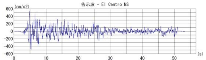
図 1 加震波形
